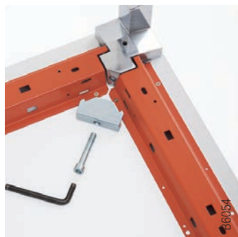
Einfach zu montieren
